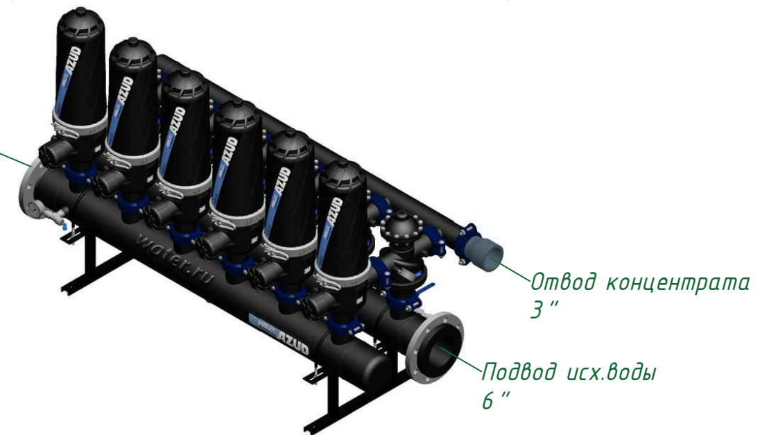
Изометрия
